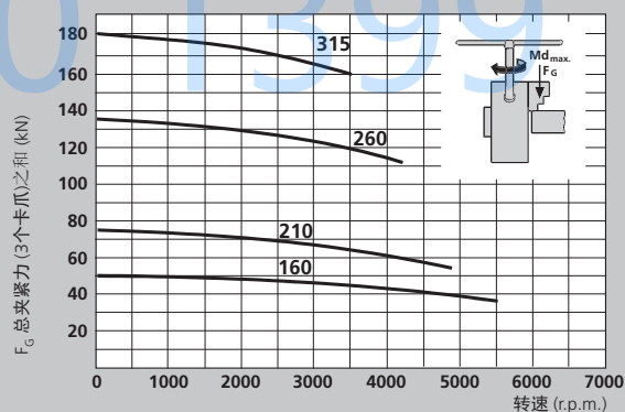
用于最高转速 平面夹紧力曲线
