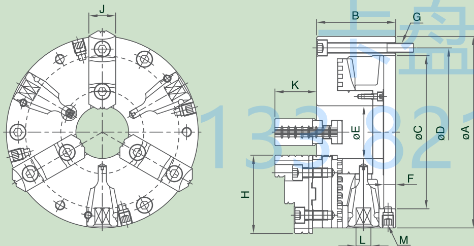
尺寸圖 » Dimensions
